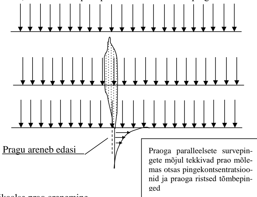
Skeem 4.6 Vertikaalse praod arenemine
