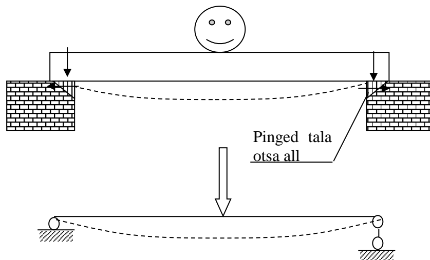
Skeem 2.1 Tala arvutusskeem
