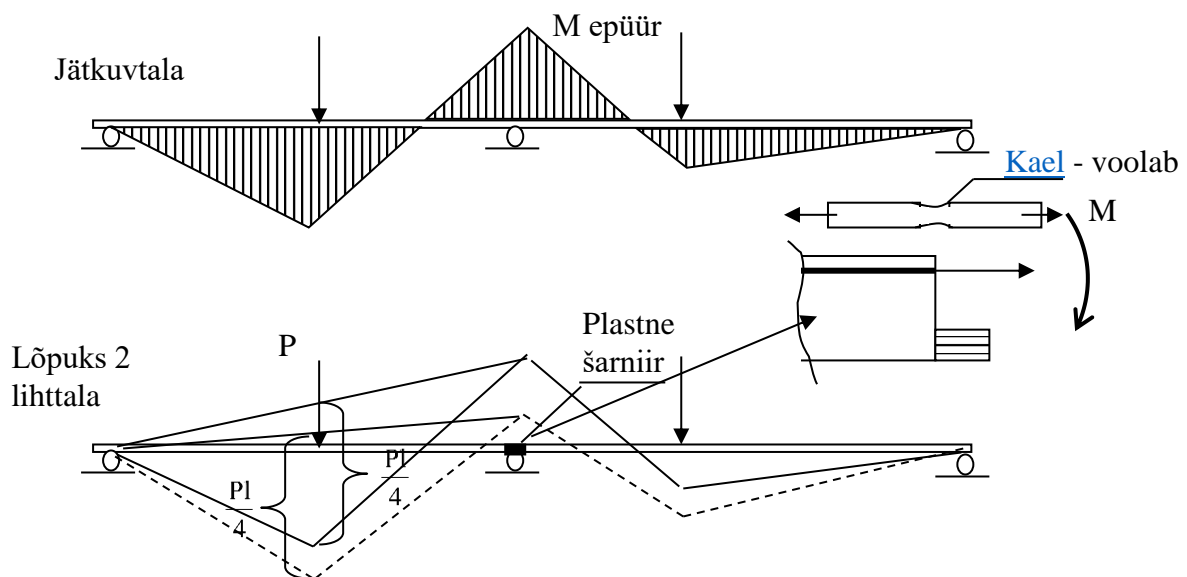
Skeem 1.3 Jõudude ümberjaotumine talas
