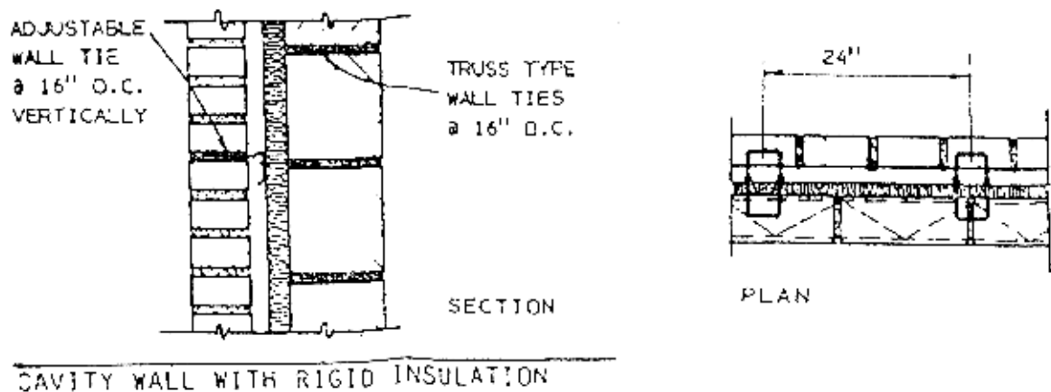
Skeem 4.14 Soojustusega sein väikeplokkidest
